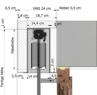
VUS-VORBAU UNTERPUTZSCHACHT
