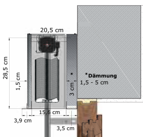
ISO-EPS-PLUS VORBAUELEMENT
