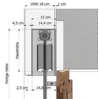
AUS-AUFSATZ UNTERPUTZSCHACHT
